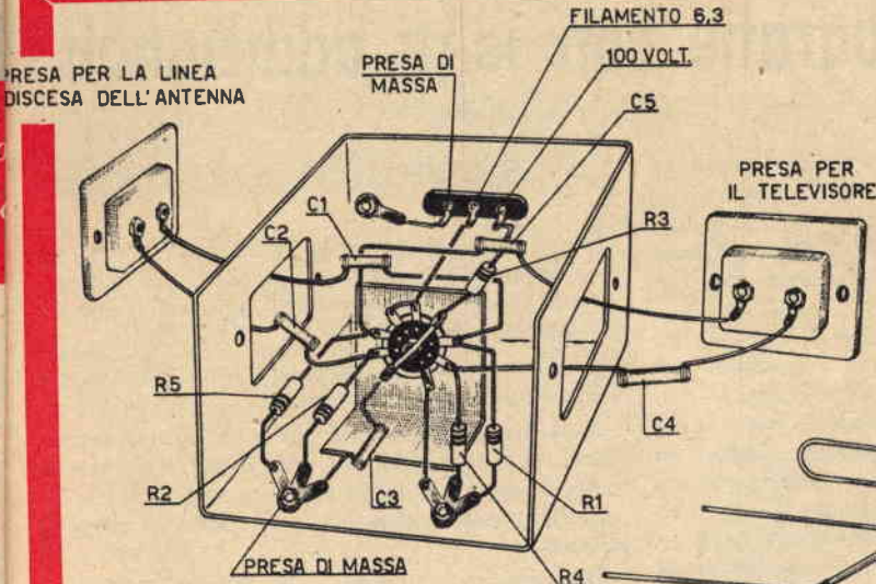
Fig. 2 - Schema pratico.
