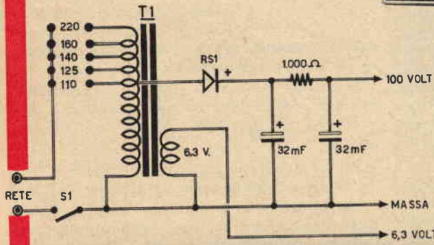
Fig. 3 - Alimentatore separato.
