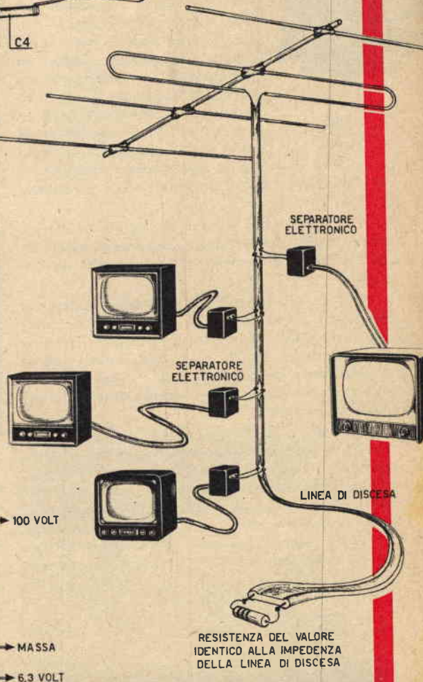
Fig. 2 - Schema pratico.
