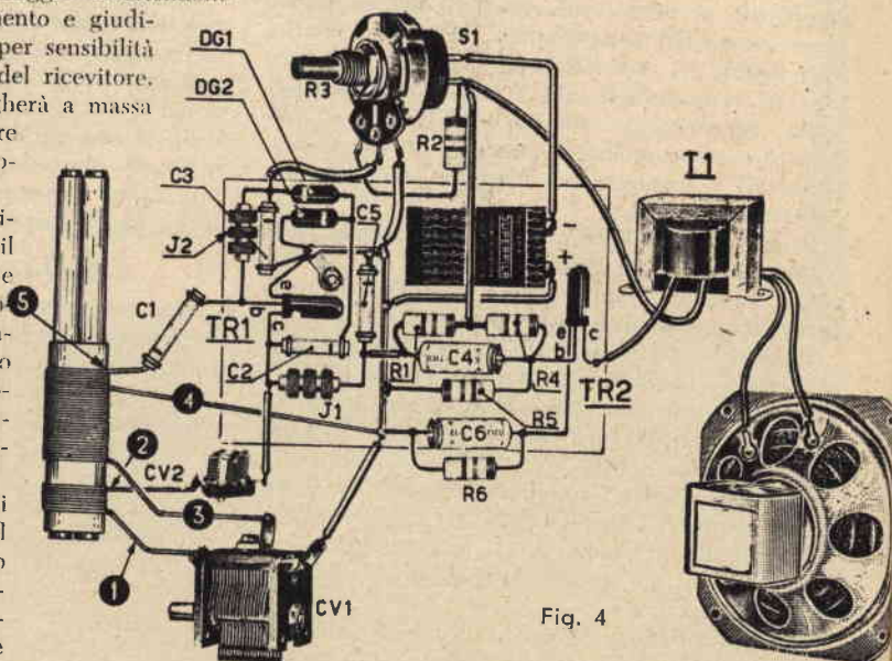
Fig. 4 - Schema pratico.
